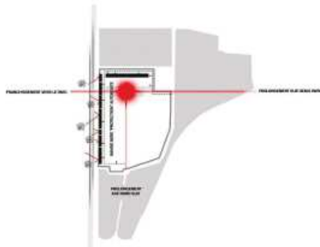
Front bât utilisé comme écran acoustique
